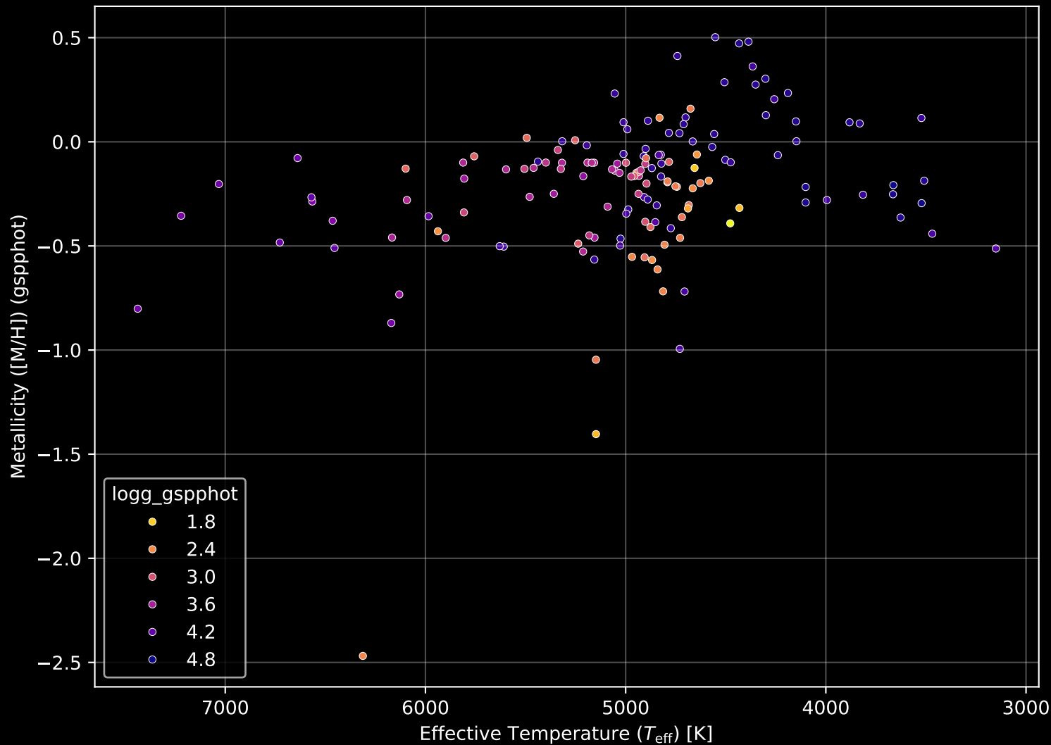
APOGEE DR17 Field: [K2_C6_316+48_btx] Stellar Population Parameters (n= 151)
