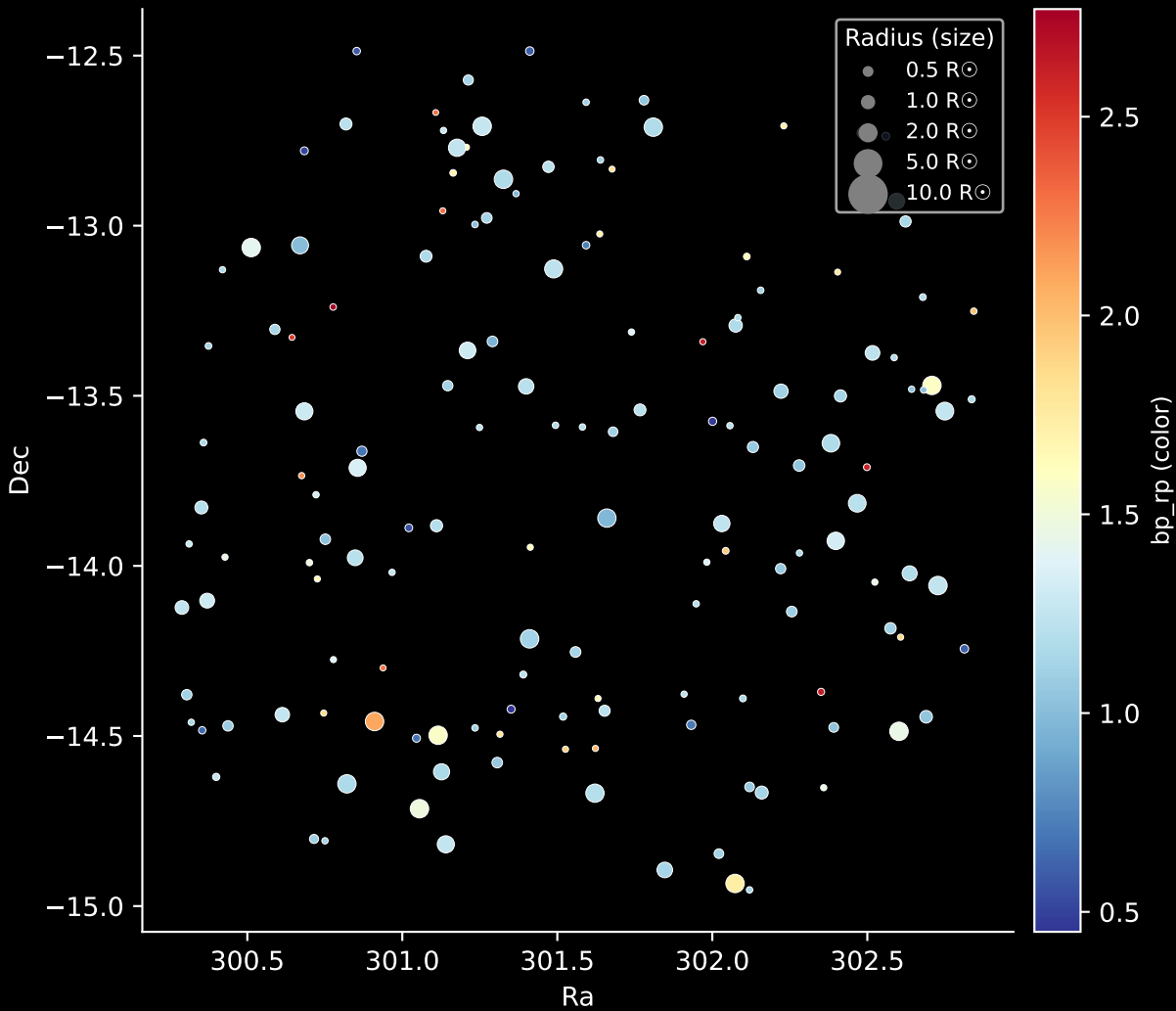
APOGEE DR17 Field: [K2_C6_316+48_btx] Stars: 151
